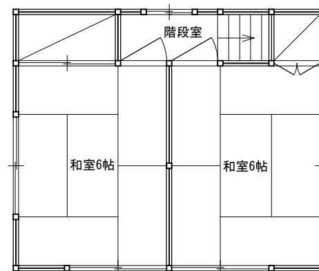
2 階 平 面 図 1 / 1 0 0
