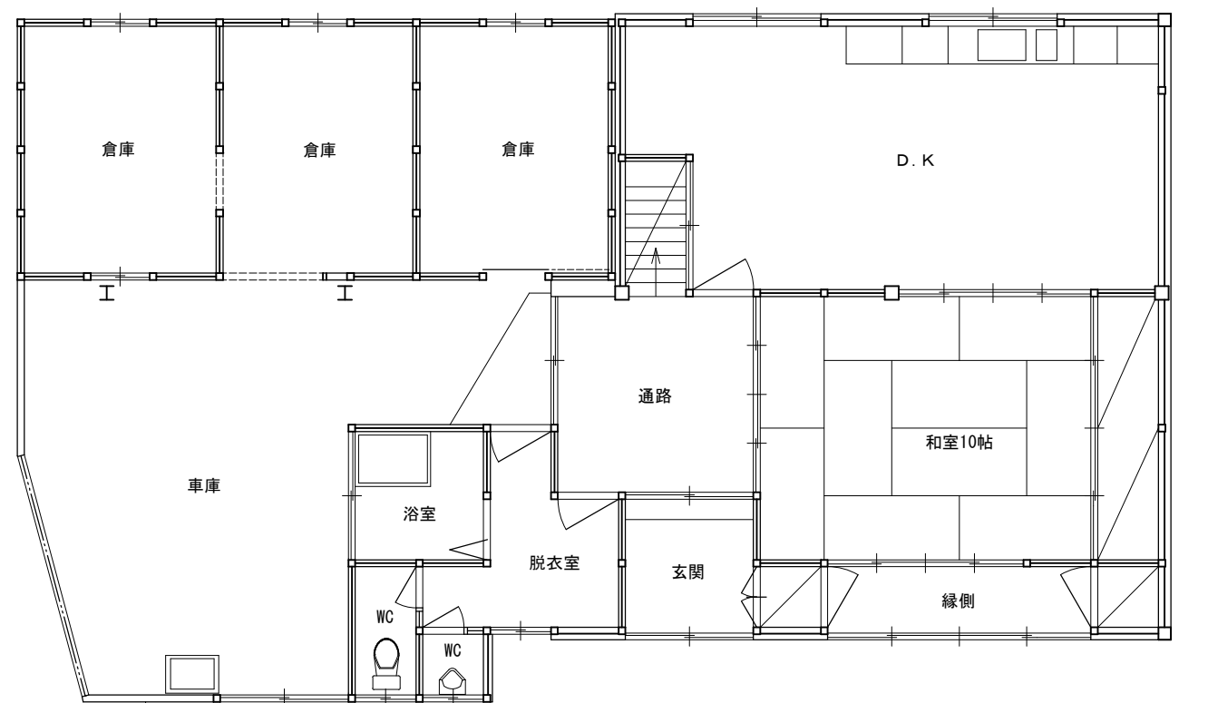
1 階 平 面 図 1/100
