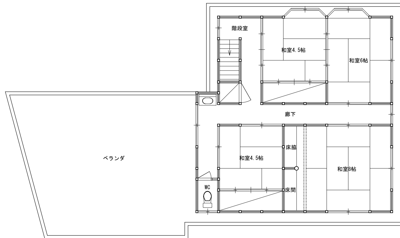
2 階 平 面 図 1/100
